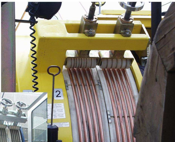
KOŁO WIELOROWKOWE
